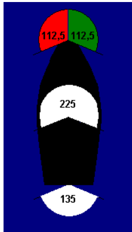
Topplicht mind. 1 Meter höher als die Seitenlichter
