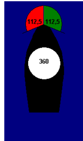
Rundumlicht mind. 1 Meter höher als die Seitenlichter
