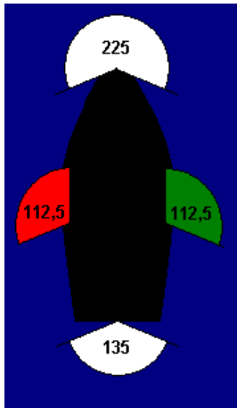
Topplicht in gleicher Höhe wie die Seitenlichter, jedoch mind. 1 Meter davor
