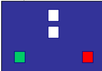
Erstes Fahrzeug: Zwei Toplichter, Seitenlichter und gelbes Hecklicht (Schlepplicht)
