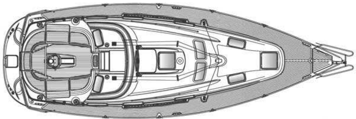
Decksplan
