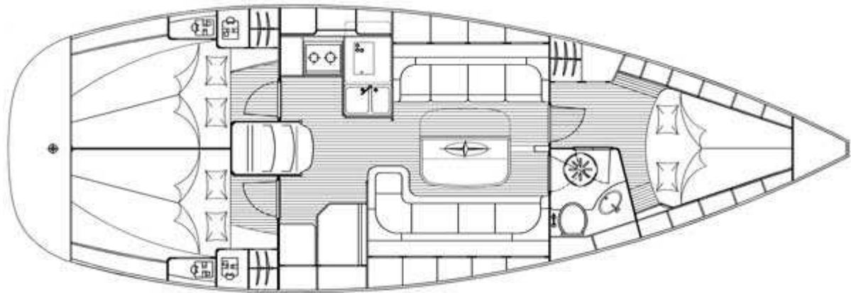
Einrichtungsplan
